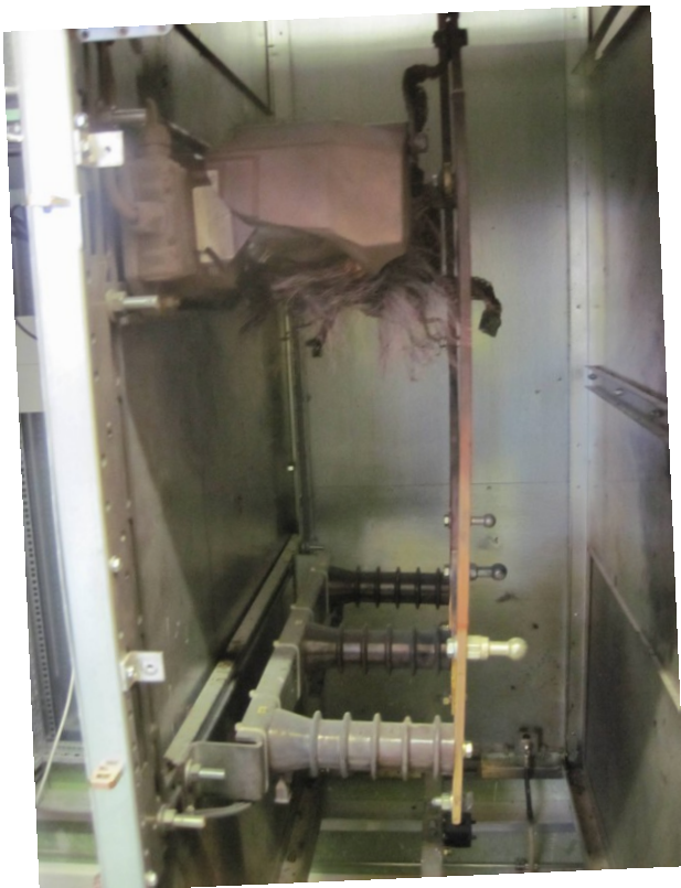
Foto: Mittelspannungszelle mit defektem Spannungswandler
